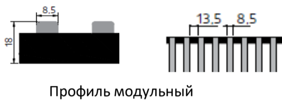
Профиль модульный
